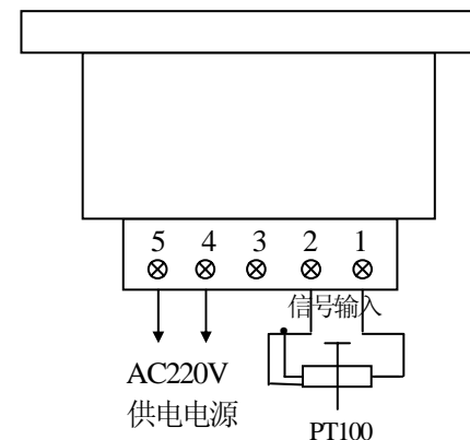
XL3000T-2 温度表交流供电输入接线图
